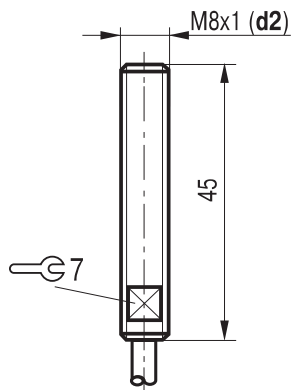
Схема монтажа
